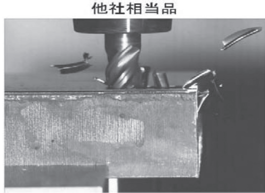
切りくずが常に溝の中に留まる傾向がある 加工途中で切りくず噛み込みも発生
