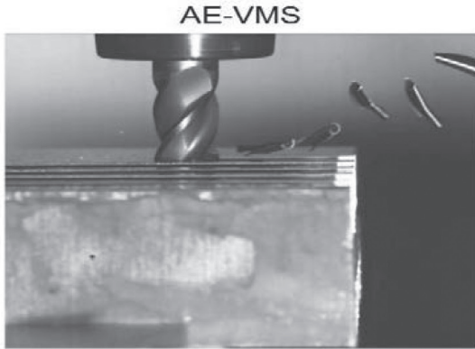
切りくずが常に溝の外に排出されている
