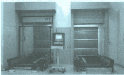
コンベア連動・門番 外部より搬入される製品・資材をコンベアに乗せたままパスルームとしてお使いいただけます。
