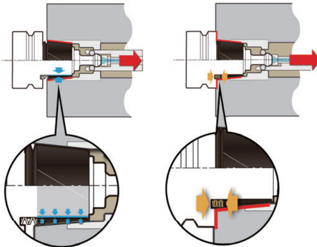
テーパコーンによる 高い密着性と振動減衰
